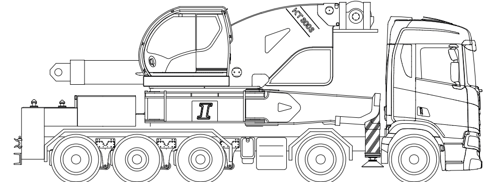
Senza braccio e stabilizzatori posteriori : peso tot. 40.000 Kg Without boom and rear outriggers : total weight 40.000 Kg.
